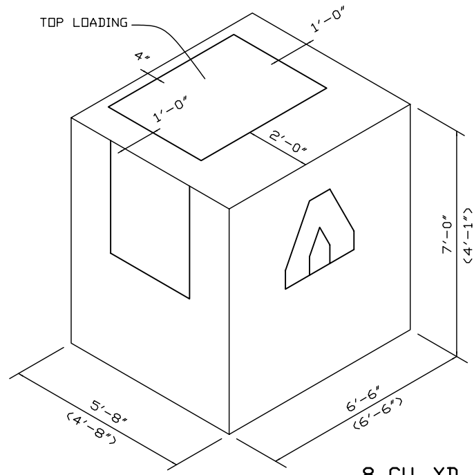
8 CU. YD. CONTAINER (4 CU. YD. CONTAINER)
